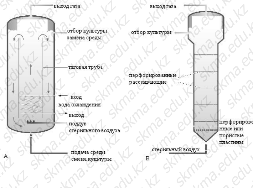
Рис.3. Ферментеры с пневматическим перемешиванием:
