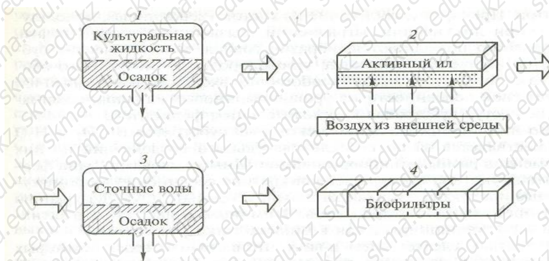
Рис. 12. Схема биологической очистки жидких отходов:
